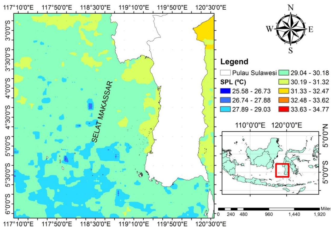
Gambar 4. Suhu Permukaan Laut (SPL) perairan Selat Makassar.
